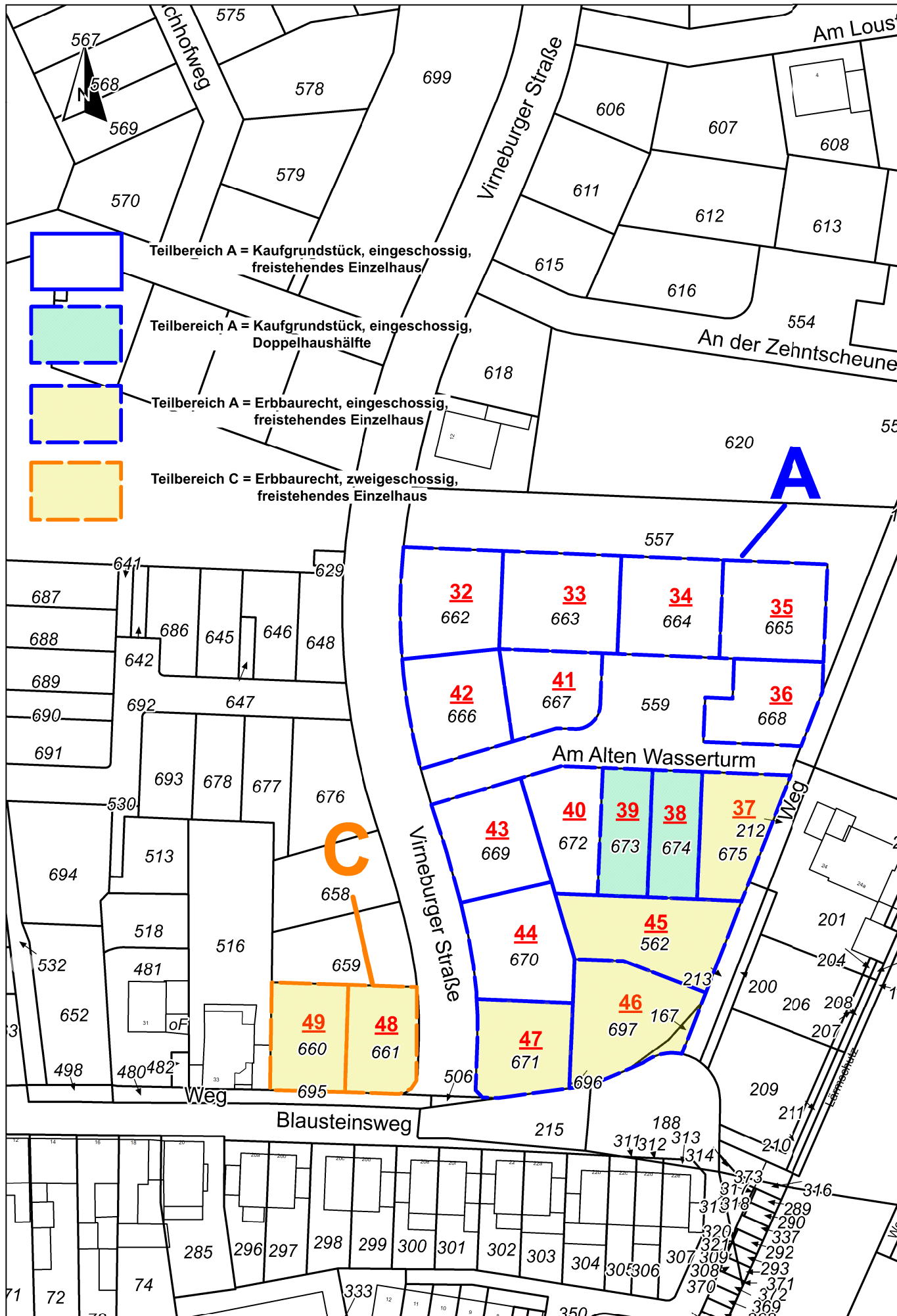
Maßstab 1:1000
